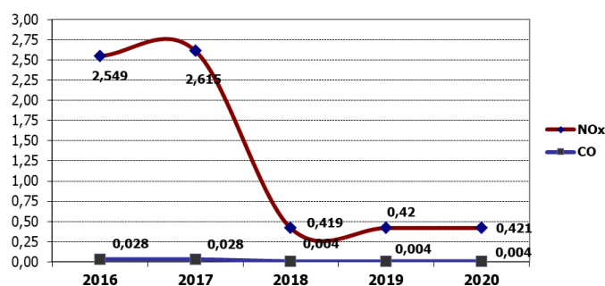
Vývoj produkce NOx a CO v období 2016-2020 (v t)
