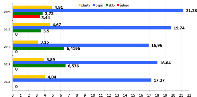
Produkce recyklovatelných odpadů 2016-2020 (v t)
